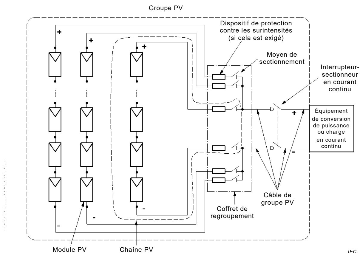
Figure A.712.2 – Groupe PV à plusieurs chaînes connectées en parallèle
